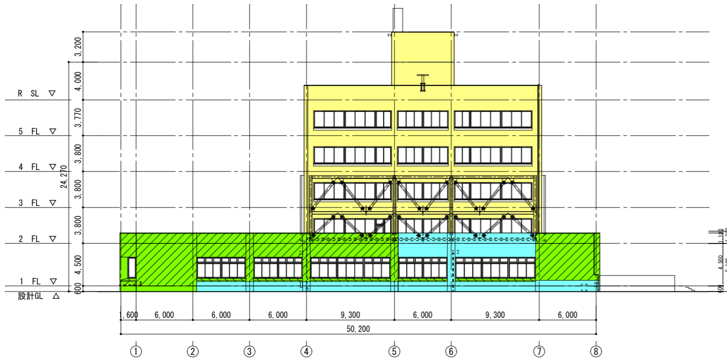
南側立面図
