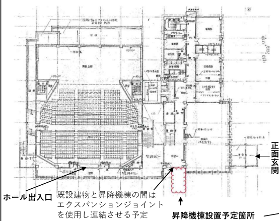
福祉会館平面図
