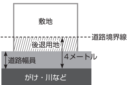
道路の後退例(2)
