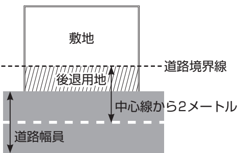
道路の後退例(1)
