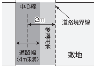
幅員4メートル未満道路の後退例1 道路の反対側が宅地などの場合は、道路中心線から2m後退
