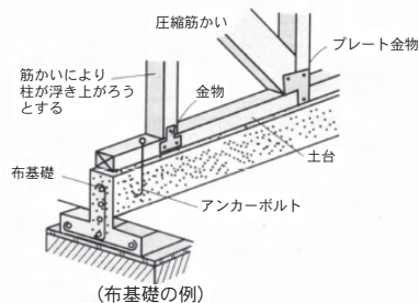
(布基礎の例)
