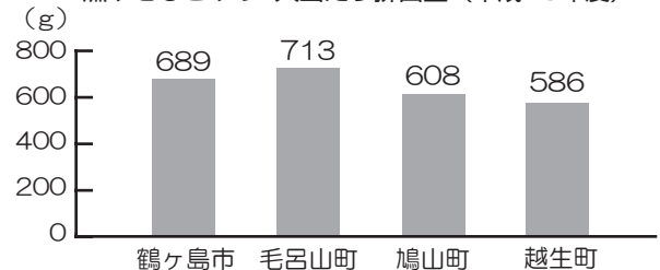
燃やせるごみの1人当たり排出量（平成19年度）
